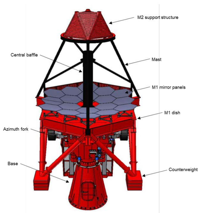
Figura 2. Modelo 3D de un telescopio de la red ASTRI. Algunos de los componentes optomecánicos se indican explícitamente.
