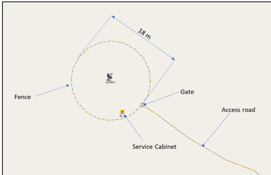
Figura 4. Propuesta de distribución del área alrededor de cada telescopio
